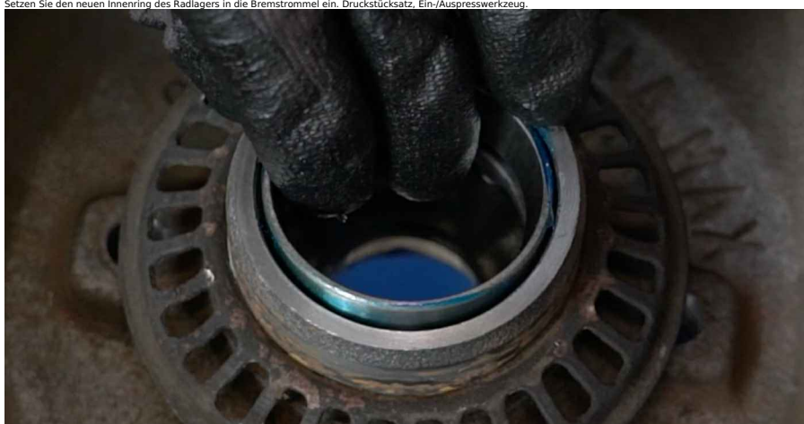
club.auto-doc.at 7-14 20 Behandeln Sie das Radnabenlager. Verwenden Sie Lagerfett.
