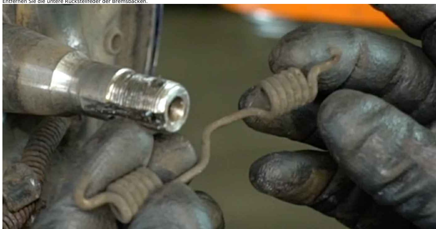
20 Trennen Sie das Handbremskabel.
