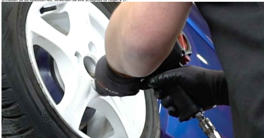
47 Schrauben Sie die Radbolzen fest. Verwenden Sie eine Schlagnuss für Felgen # 17.
