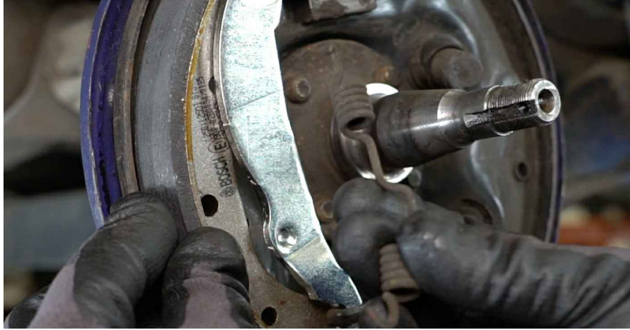
25 Bauen Sie die untere Rückstellfeder ein.
