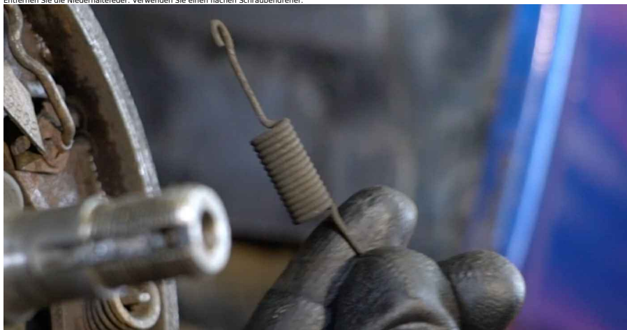
16 Entfernen Sie die Halterung der Trommelbremsbacken. Verwenden Sie ein Werkzeug für Bremsträgerfedern.
