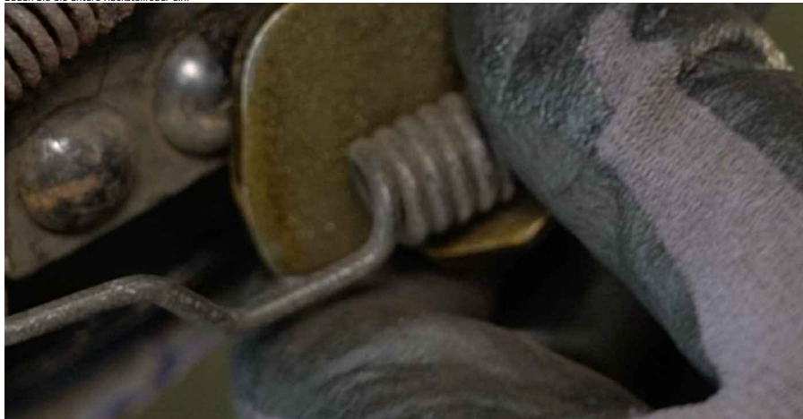
38 Installieren Sie die Halterung der Trommelbremsbacken. Verwenden Sie ein Werkzeug für Bremsträgerfedern.
